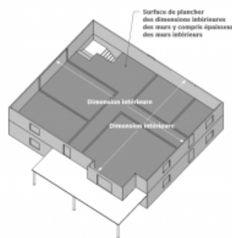
Surface de plancher finale de l'étage
