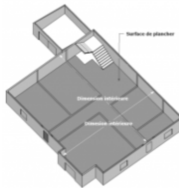
Surface de plancher finale du rez-de-chaussée
